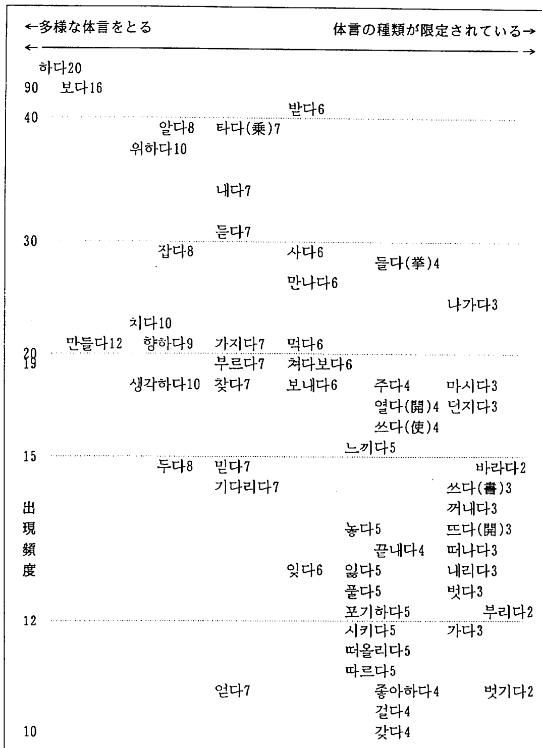
【図】用言の出現頻度と-을格の体言範疇の多様性による用言の分布 (語彙の横の数字は体言分類の種類数を示す)
